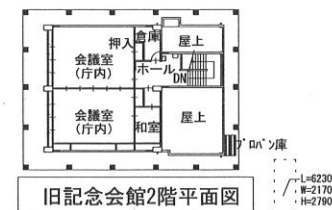
旧記念会館2階平面図
